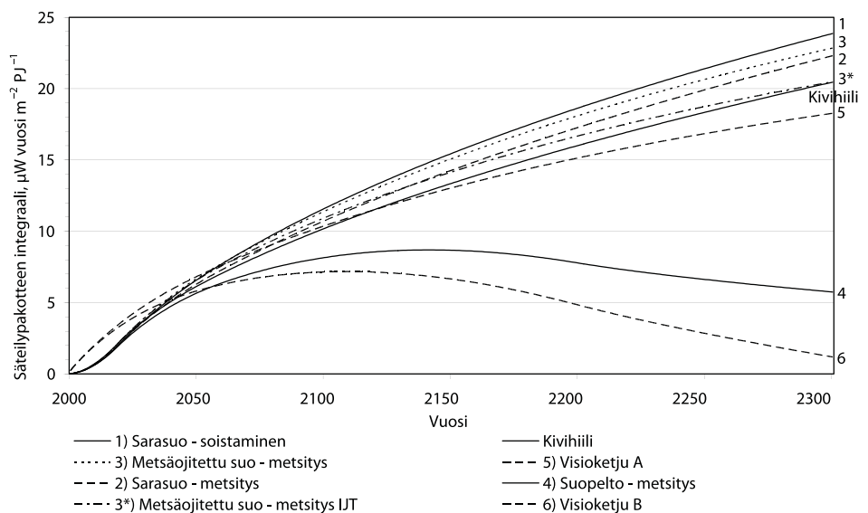
Kuva 29. Eri turvetuotantoketjujen ja kivihiihen aiheuttama kumulatiivinen säteilypakote ajan funktiona tuotettua 1 PJ energia-määrää kohti. Säteilypakoteintegraali esitetään maapallon pinta-alaa kohden. Ketju 3* kuvaa tilannetta, jossa jäännösturve on kerätty pois kokonaan (ilman jäännösturvetta, IJT).
