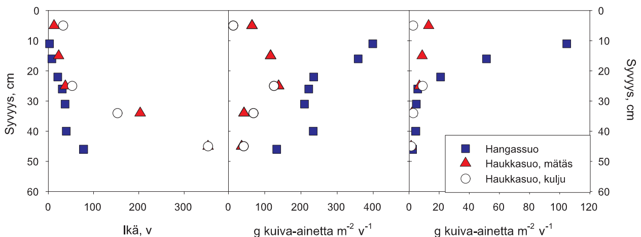
Kuva 6. Turpeen ikä, turpeen näennäiskertymä ja jäljellä oleva kuiva-aineen määrä näytteen ikään suhteutettuna eri syvyyksillä Hangas- ja Haukkasuon tutkimusalueita. Määttävät ovat keidasrämeen kuivia pintoja ja kuljut märkiä pintoja. Kuiva-aineesta noin 40–50 % on hiiltä.
