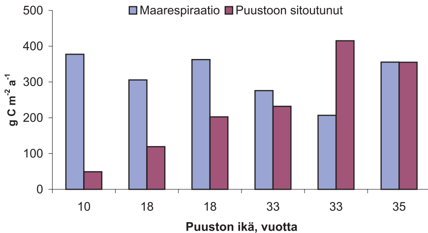
Kuva 18. Metsitettyjen peltokohdeiden vuotuinen heterotrofinen maahengitys ja puustoon mitausjakson aikana vuosittain sitoutuneen hiilen määrä.
