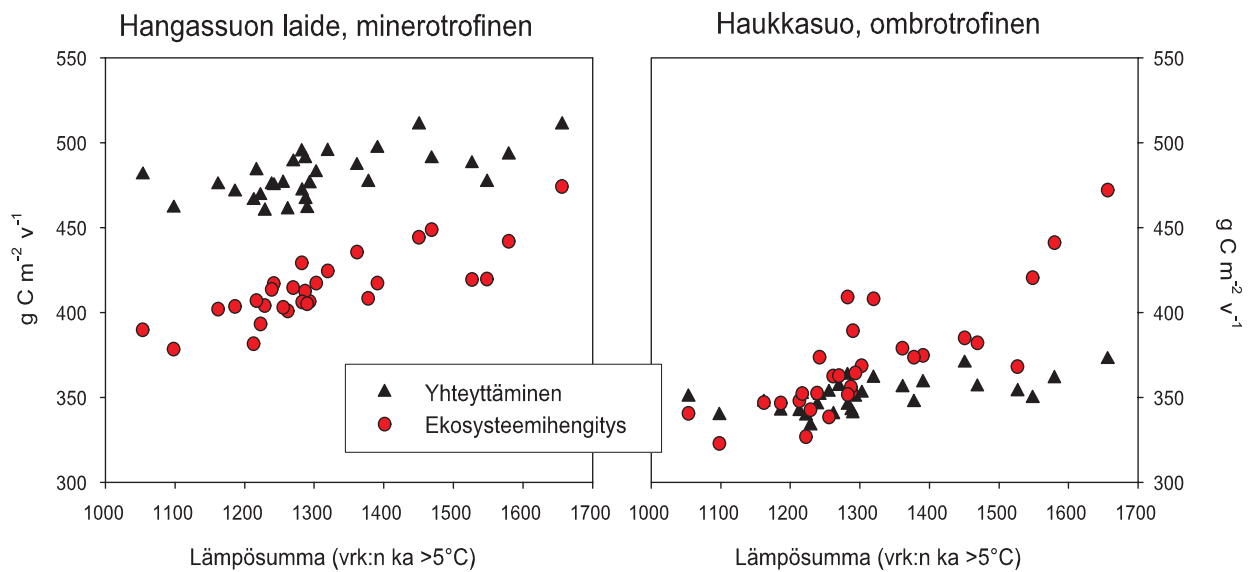
Kuva 3. Hangas- ja Haukkasuon simuloitujen hiilidioksidivaihdot olivat sitä suurempia mitä suurempi oli vuotuinen lämpösumma. Lämpösumma perustuu vuorokauden keskilämpötilaan ja siinä lasketaan yhteen ne lämpöasteet, jotka ylittävät 5 °C. Simuloitujen vuosien sääolojen vaihtelu vastasi vuosien 1961–1990 vaihtelua Anjalankoskella.
