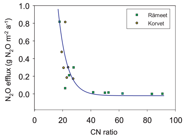
Kuva 11. Typpioksiduulipäästöt metsäojitetuilta soilta hiilityypisuhteen funktiona.
