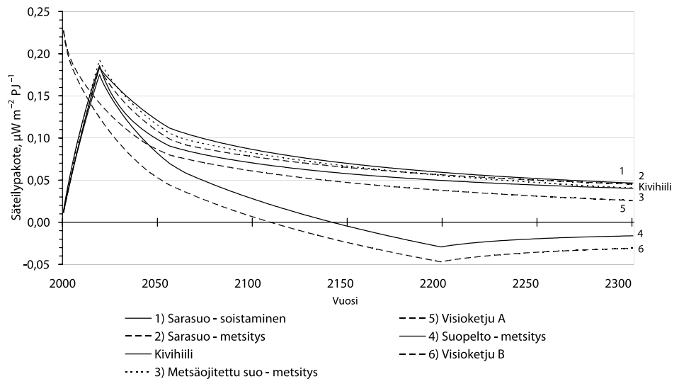
Kuva 28. Eri turvetuotantoketjujen sekä hiilen tuotantoketjun aiheuttama hetkittäinen säteilypakote ajan funktiona. Säteilypakote esitetään maapallon pinta-alaa kohden.
