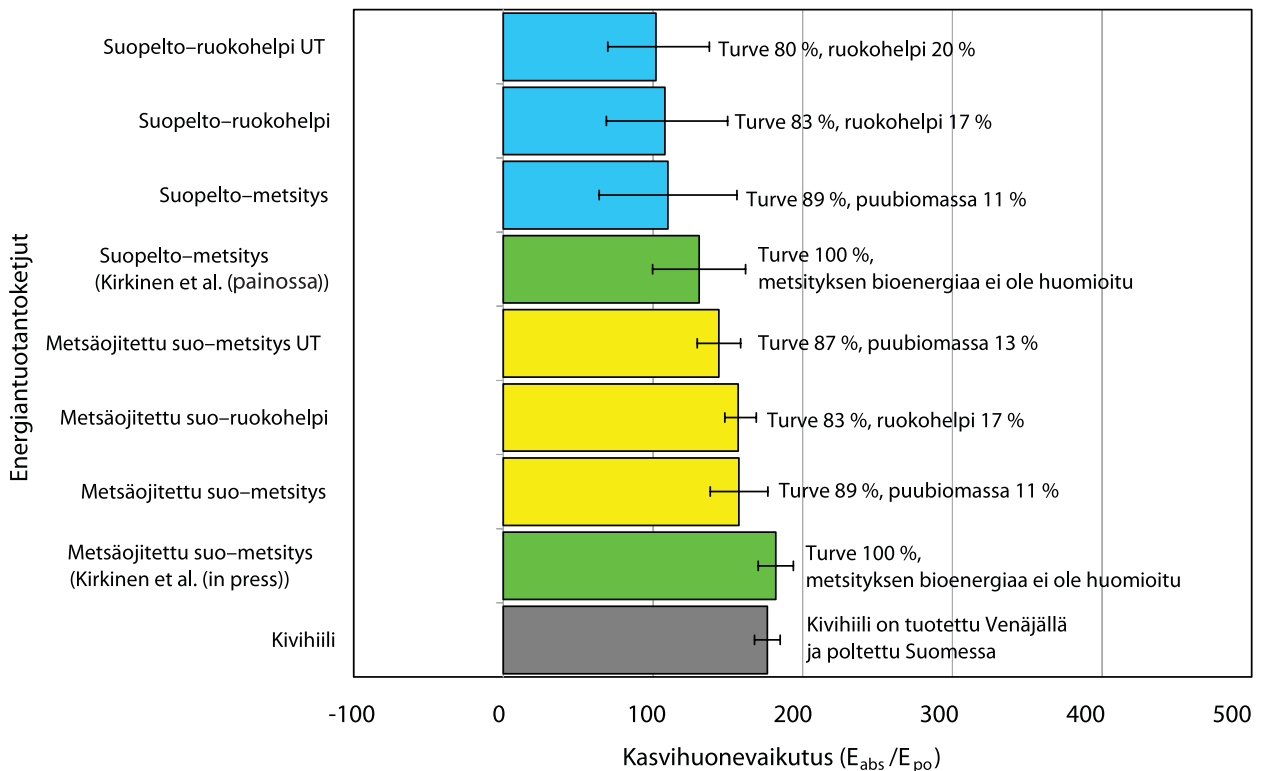
Kuva 30. Eri energiantuotantoketjujen kasvihuonevaikutus sadan vuoden tarkasteluajalla turvemaankäyttöskenaarioissa ja kivihiiliskenaarioissa. Palkit kuvaavat kunkin ketjun kasvihuonevaikutusta ja vaakasuorat janat kuvaavat vaikutuksen epävarmuutta. Keltaisissa ja sinisissä palkeissa on esitetty, kuinka paljon kyseisissä ketjuissa on tuotettu energiaa turpeella ja kuinka paljon uusiutuvalla bioenergialla. Kasvihuonevaikutus ( E_{abs}/E_{po} ) on elinkaaren päästöjen ja nieluun aiheuttama kumulatiivinen säteilypakote sadassa vuodessa jaettuna polttoaineen energialla (UT= uusi turpeen tuotantomenetelmä).
