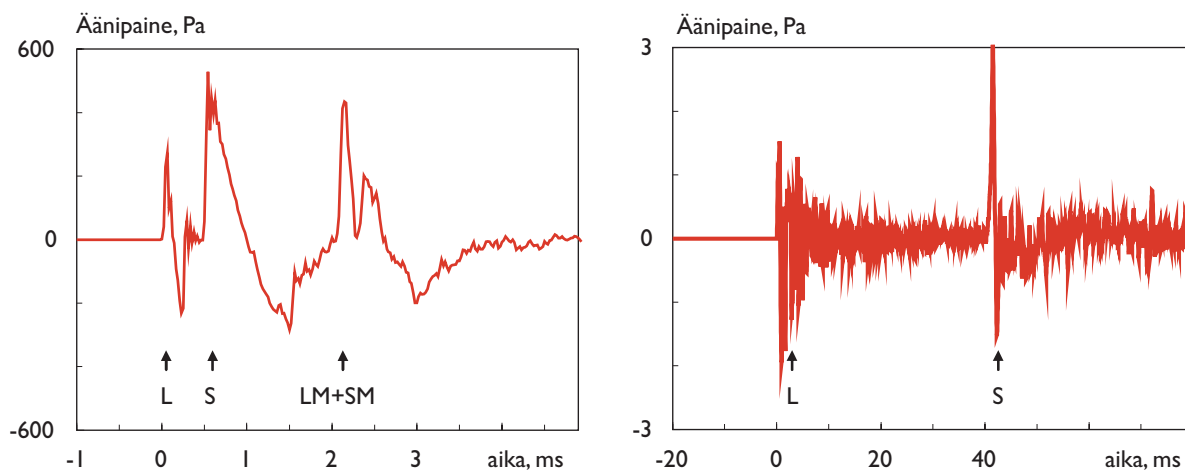
Kuva H8. Rynnäkkökiväärin laukaus etäisyydellä 10 m (vasen) ja 300 m (oikea); L: luotiääni, S: suupamaus, LM+SM: luotiäänen ja suupamauksen maaheijastus. (Kuvien aika-akselit erisuuret.)
