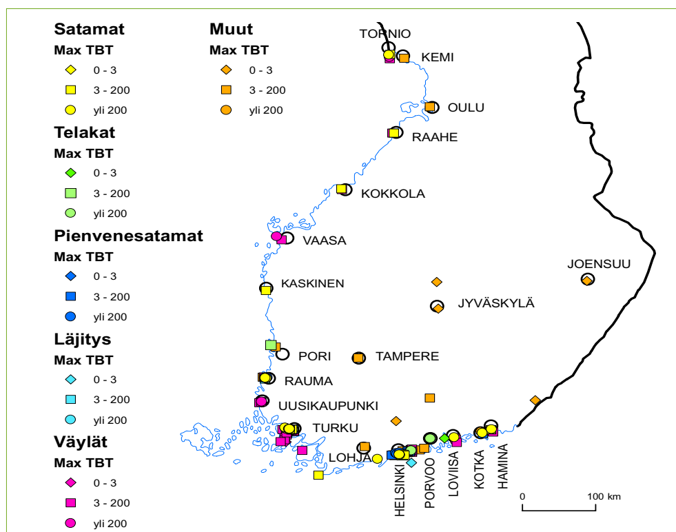
Kuva 4. Suomessa vuosina 1998 - 2005 tehtyjen TBT-tutkimusten maksimipitoisuudet (µg/kg normalisoituina) pilaavan toiminnon mukaan jaoteltuna.
