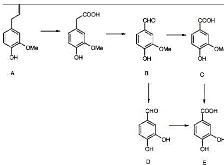
Kuva 4. Eugenolin otsonoinnin ensimmäiset vaiheet (Amat ym. 2005).
