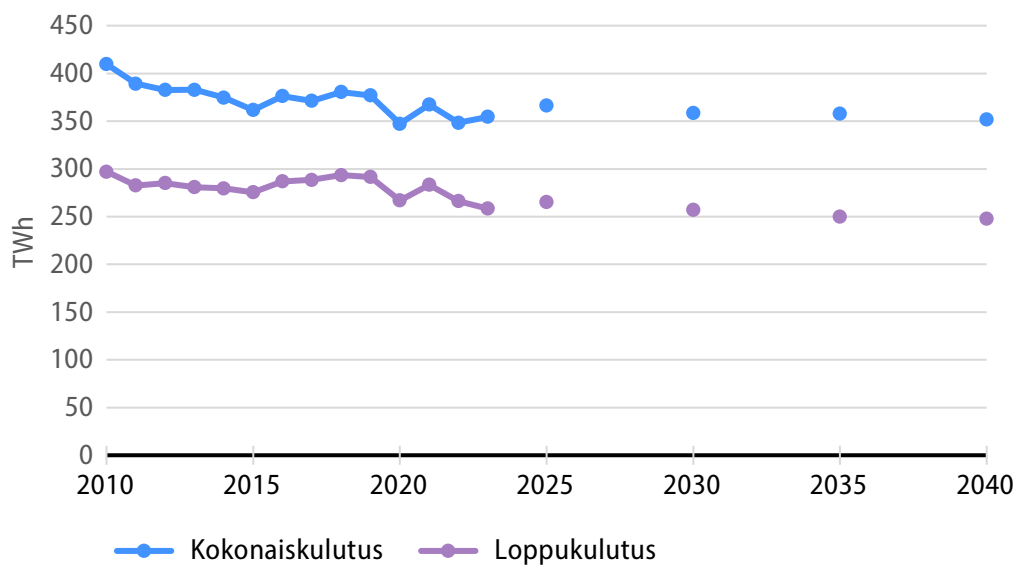
Kuvio 7. EU:n Energiatohokkuusdirektiivin mukaisesti laskettujen energian kokonais- ja loppukulutuksen tunnuslukujen historia 2010–2023 sekä kehitysarvio vuoteen 2040 asti.
